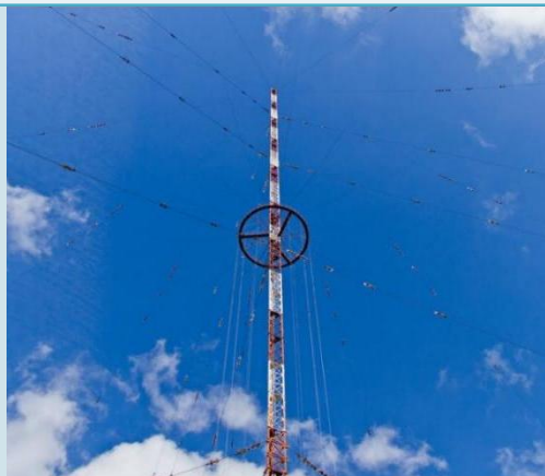
Антенна Броварского радиопередающего центра высотой 259,5 м.
